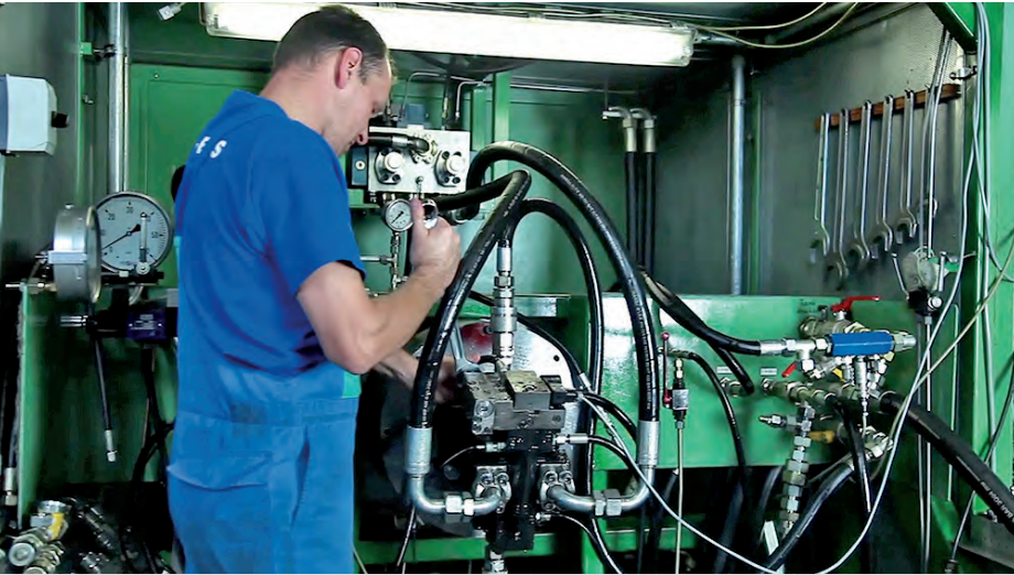
Prüfstände für offenen und geschlossenen Kreis
