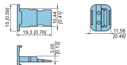
Wedgelock
