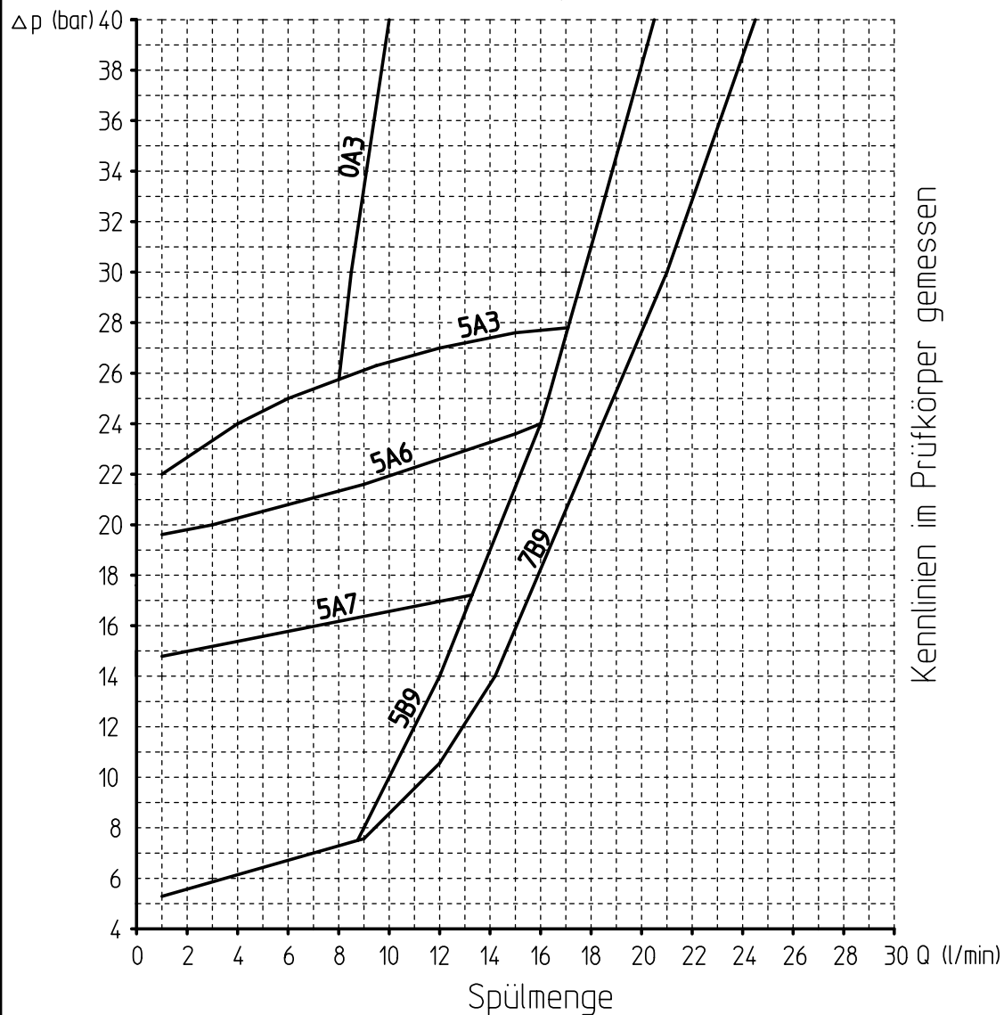
Kennlinien Spül-DBV
